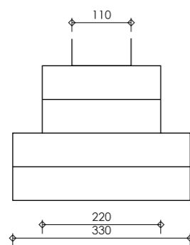
doorsnede 2
