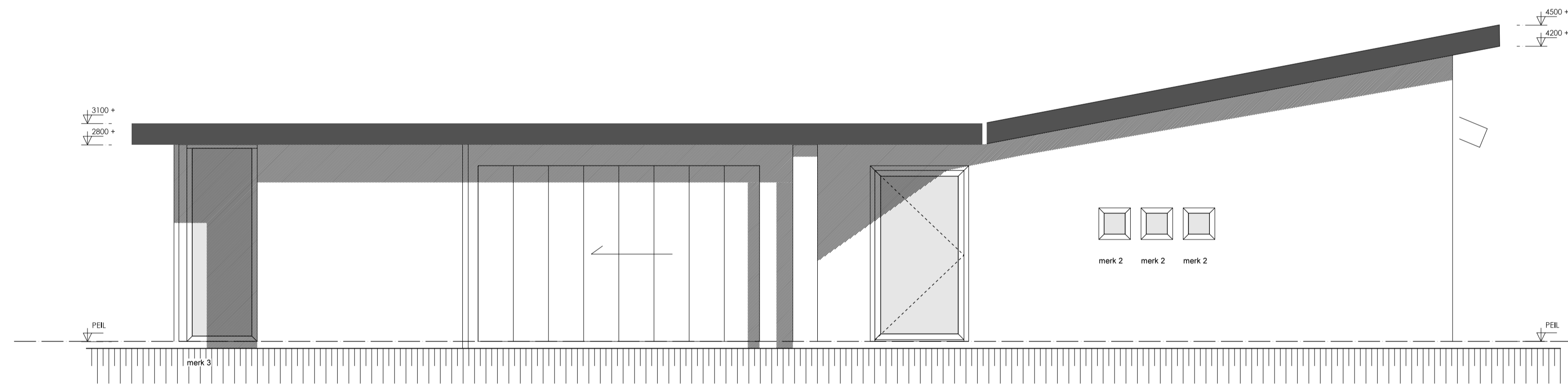
westgevel
